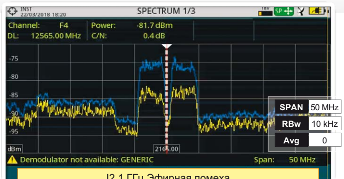
12.1 ГГц Эфирная помета с базовой станции мобильного телефона
