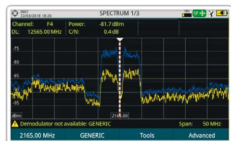
Interferencia de 2,1 GHz en banda terrestre desde una estación de telefonía móvil
