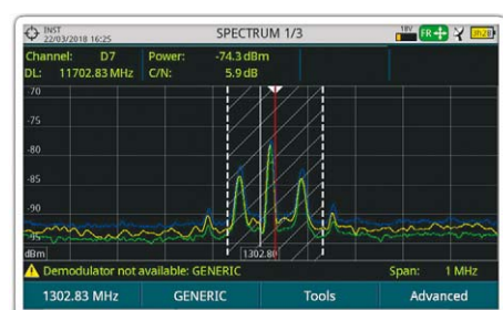
Beacon satélite con Max/Min Hold
