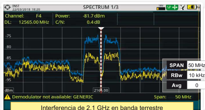
Interferencia de 2,1 GHz en banda terrestre desde una estación de telefonía móvil
