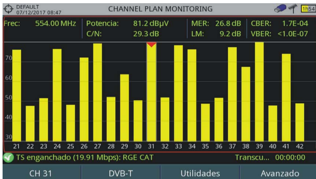
Figura 69. Monitorización de Canalización
