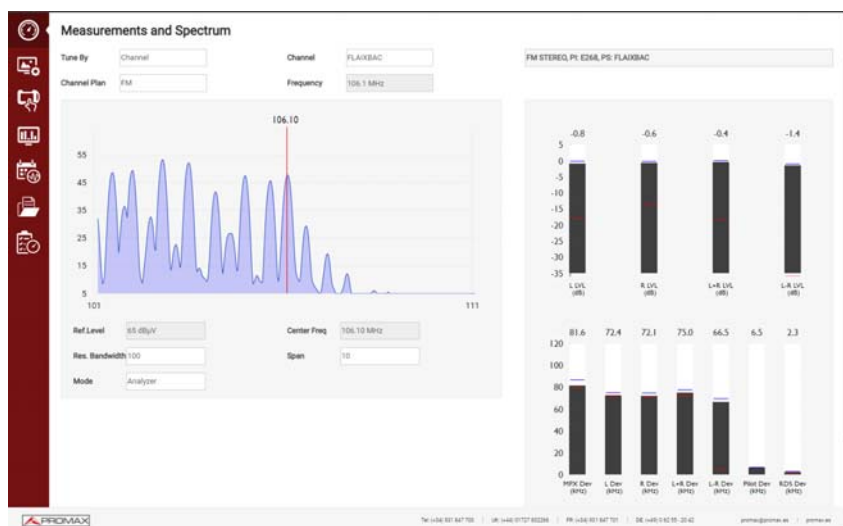
Figura 178. Medidas y Espectro de FM Avanzado
