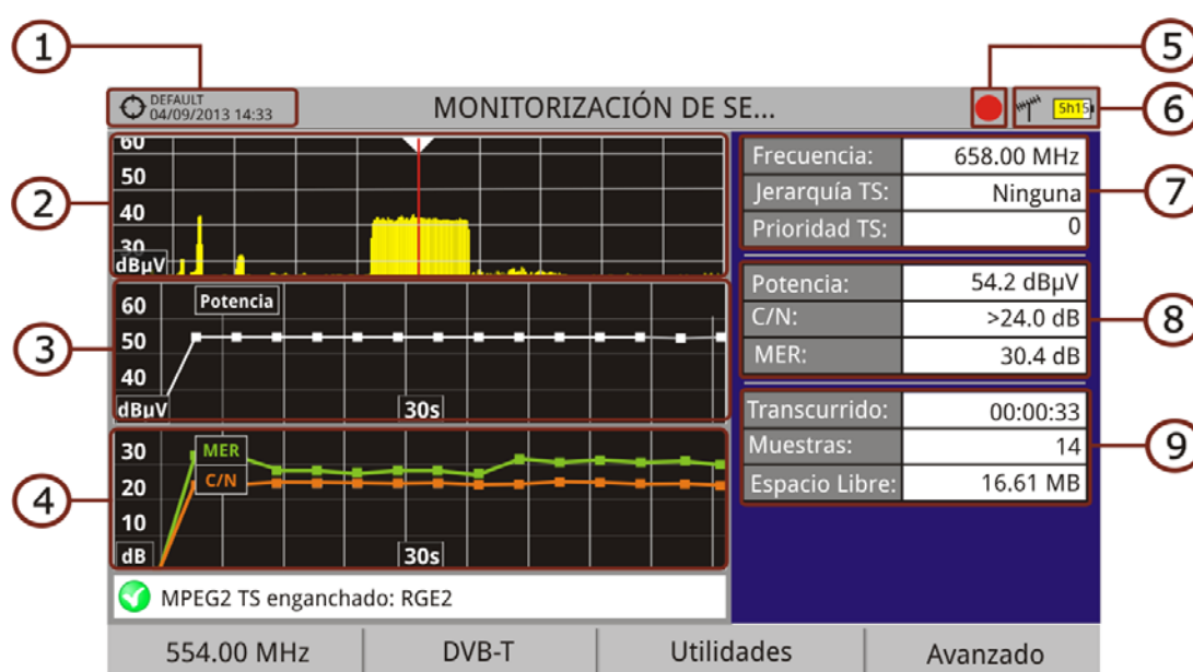
Figura 68. Monitorización de Canal Único
