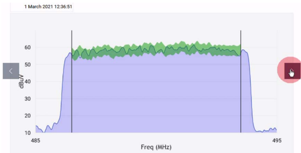
Figura 147. Gráfica de Espectro de Monitorización (detección por Desviación)
