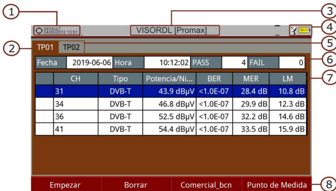
Figura 87. Visor de Datos de Canalización.
