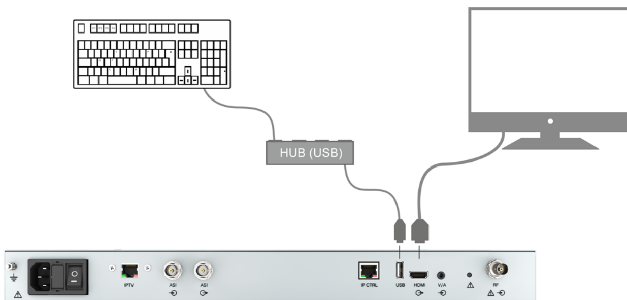
Figura 6. Conexión en Modo Local
