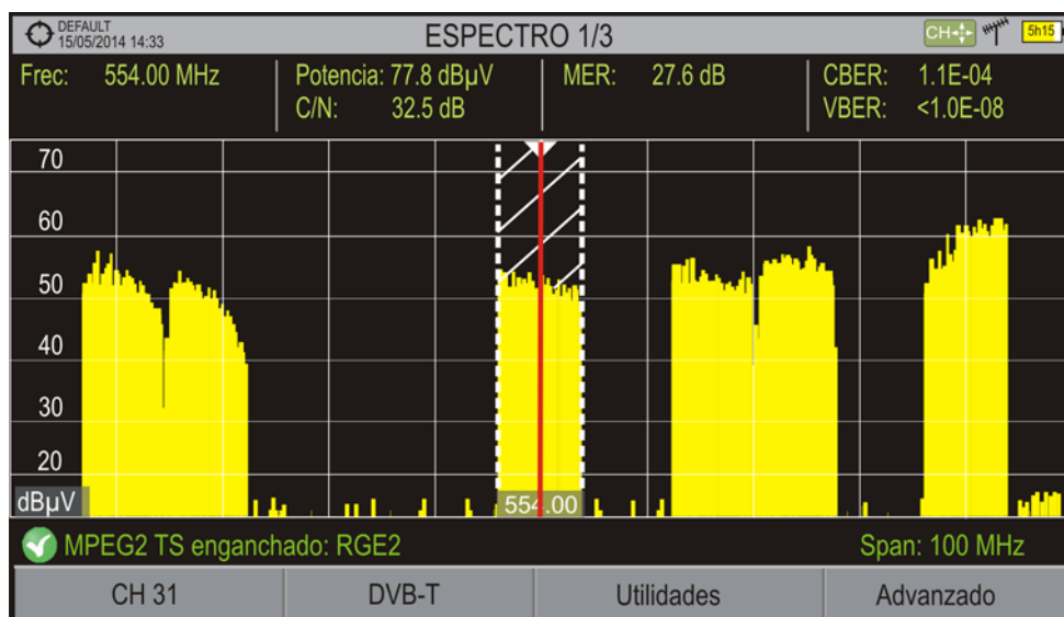
Figura 12. Pantalla inicial (canal enganchado).
