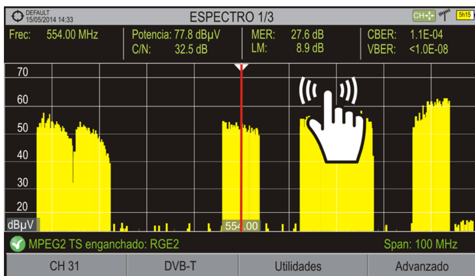
Figura 13. Pulsar sobre la nueva frecuencia.
