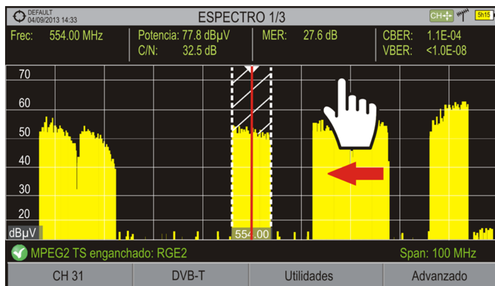
Figura 15. Pulsar y arrastrar para desplazarse
