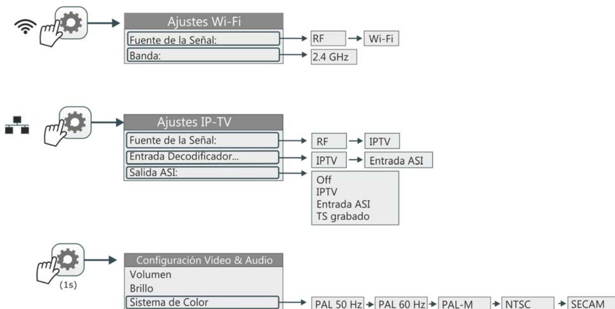
Figura 42. Menús de Ajuste para Fuente de Señal WiFi e IPTV*.
