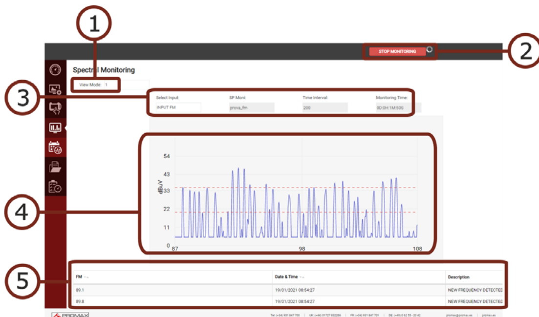
Figura 143. Monitorización en funcionamiento (detección FM)
