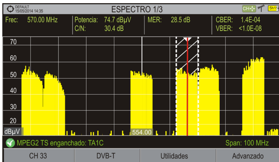
Figura 14. El cursor se desplaza a la nueva frecuencia.
