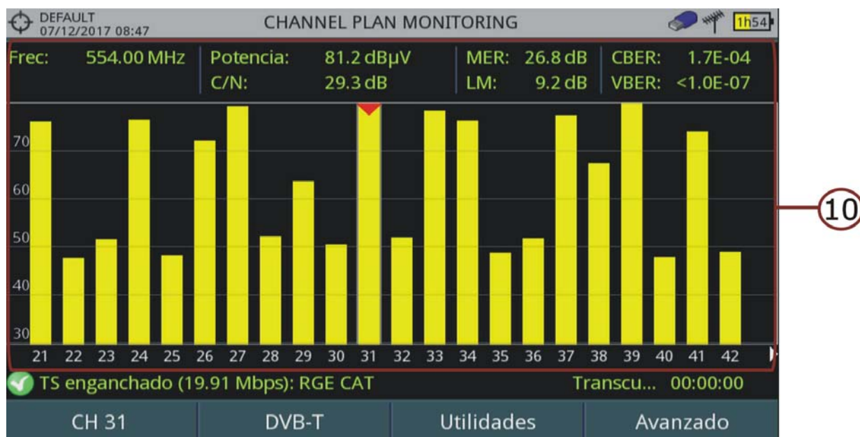
Figura 75. Cobertura de Señal de Canalización
