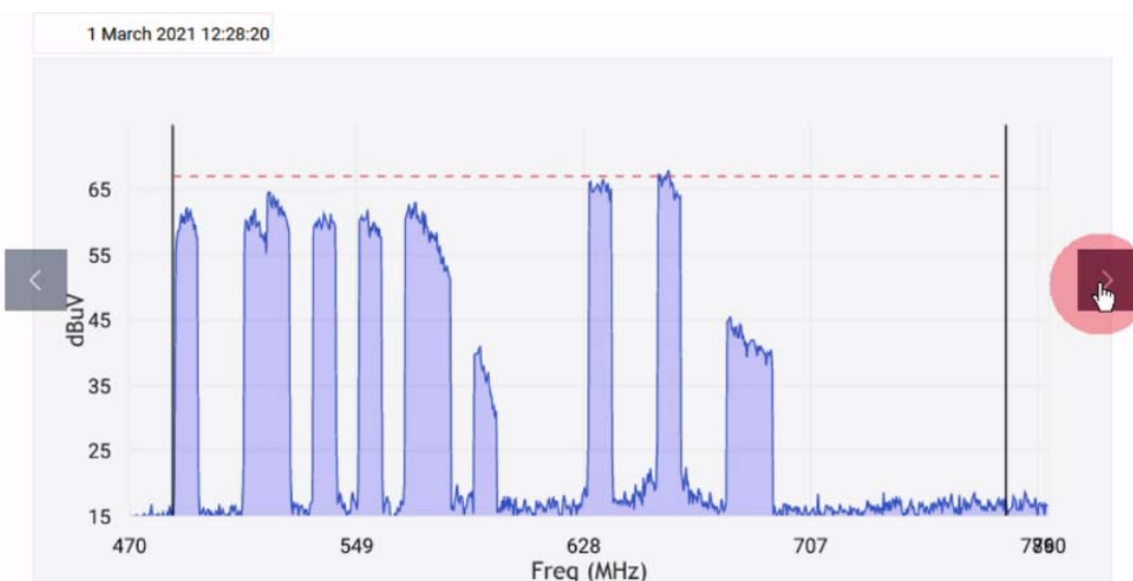
Figura 146. Gráfica de Espectro de Monitorización (detección por Max/Min)
