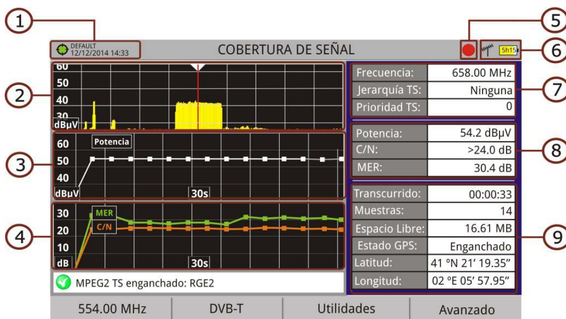
Figura 74. Cobertura de Señal de Canal Único
