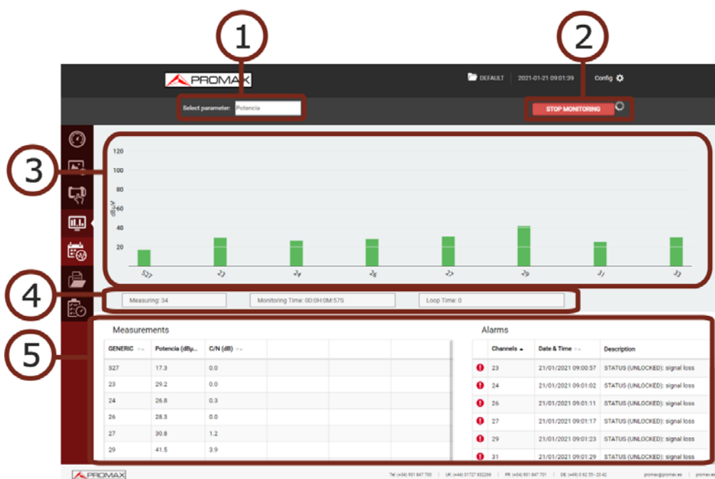
Figura 135. Monitorización en funcionamiento
