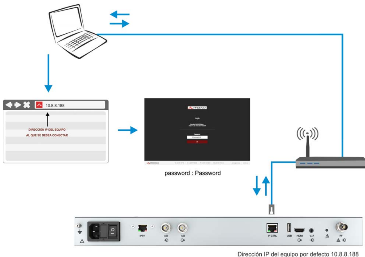
Figura 7. Conexión en Modo Remoto
