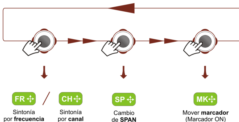
Figura 25. Funciones del Joystick en modo ANALIZADOR DE ESPECTROS.
