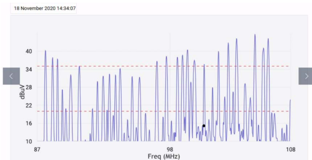
Figura 145. Gráfica de Espectro de Monitorización (detección por FM)
