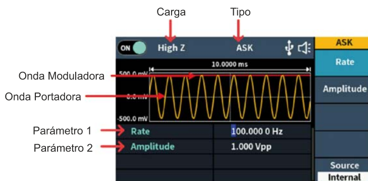
Figura 55-18: Interfaz de usuario ASK
