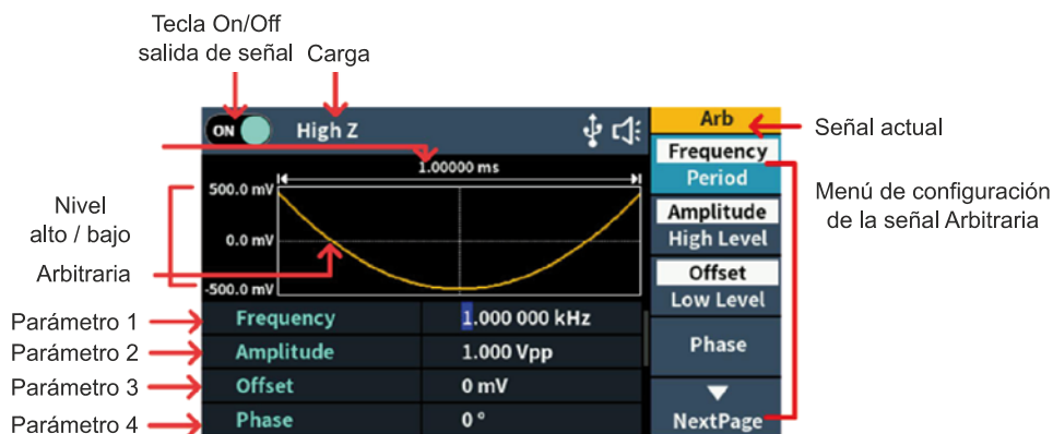
Figura 5-9: Interfaz de forma de onda Arbitraria
