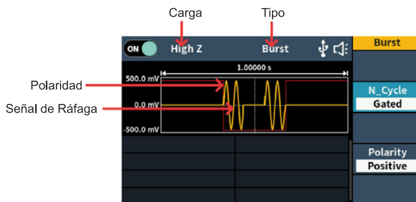
Figura 5-12: Interfaz de usuario de Ráfaga por Compuerta
