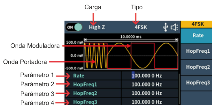
Figura 5-22: Interfaz de usuario de 4FSK
