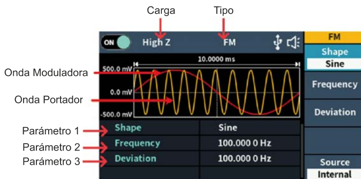
Figura 5-15 interfaz de usuario FM
