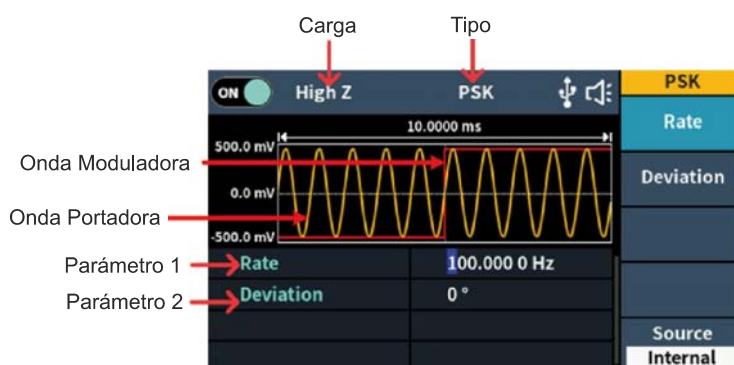
Figura 5-19: Interfaz de usuario PSK
