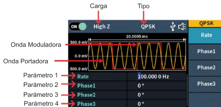
Figura 5-24: Interfaz de usuario de QPSK
