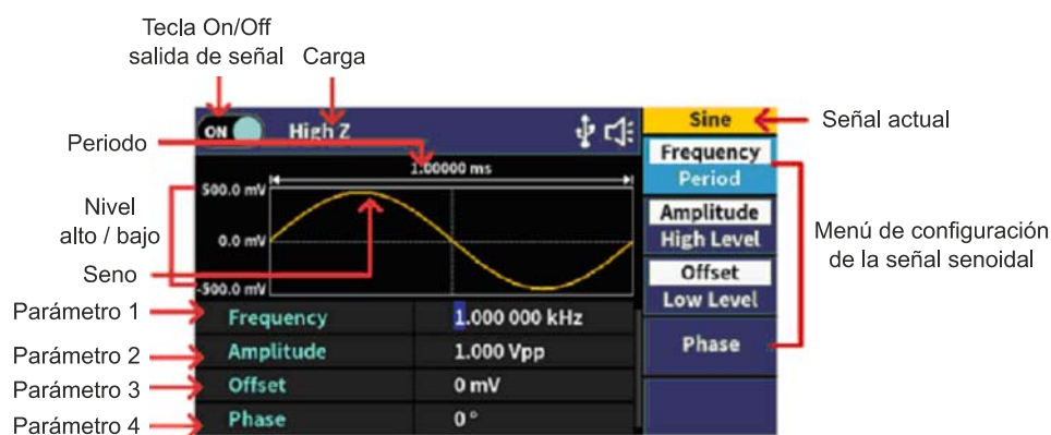
Figura 5-2: Interfaz de usuario de la onda senoidal
