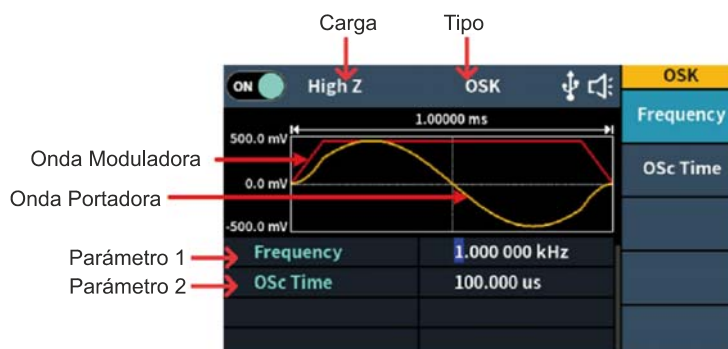
Figura 5-25: Interfaz de usuario de OSK
