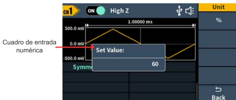
Figura 5-6: Ajustar la simetría de la forma de onda
