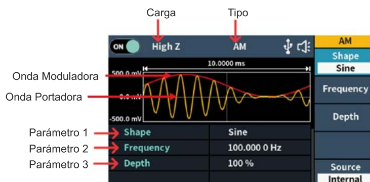
Figura 5-13: Interfaz de usuario de AM
