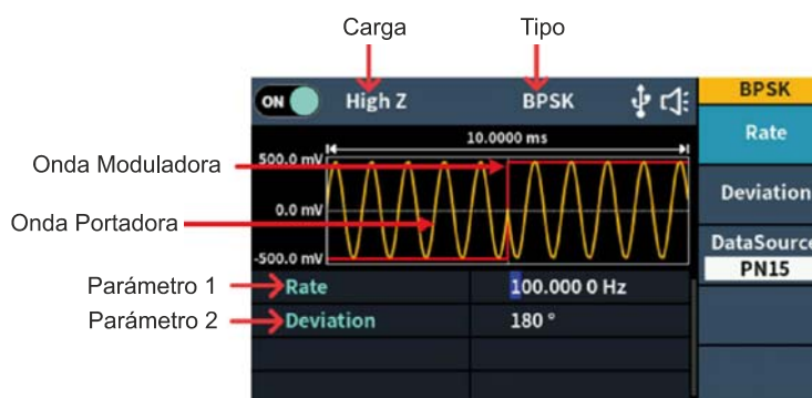
Figura 5- 23: Interfaz de usuario BPSK
