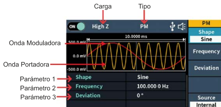
Figura 5-16: Interfaz de usuario de PM
