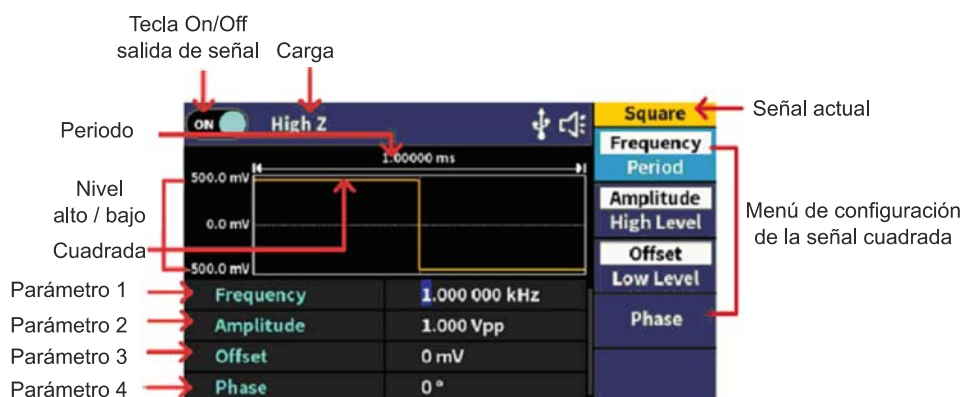
Figura 5-4: Interfaz de usuario de la onda cuadrada
