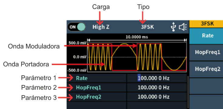
Figura 5-21: Interfaz de usuario de 3FSK
