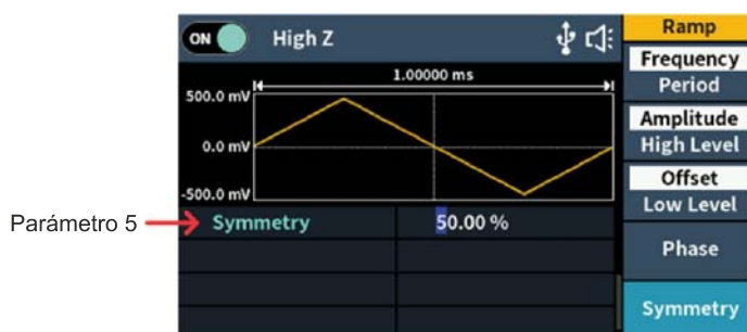
Figura 5-5: Interfaz de usuario de la onda rampa
