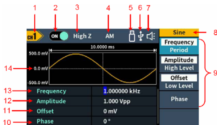
Figura 4-3: Interfaz de usuario
