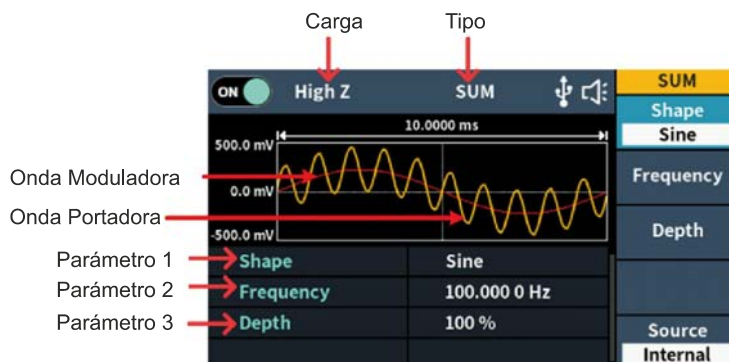
Figura 5-26: Interfaz de usuario de SUM
