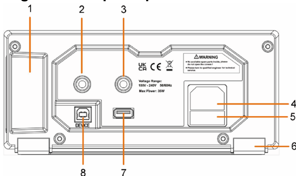
Figura 4-2: Vista general del panel posterior
