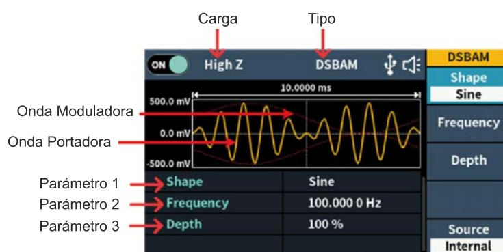
Figura 5-14: Interfaz de usuario de DSBAM
