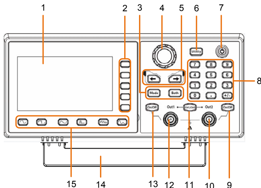
Figura 4-1: Vista general del panel frontal
