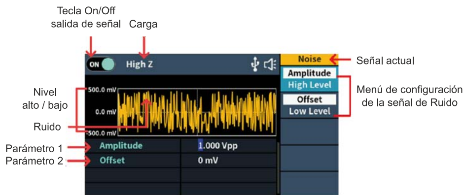
Figura 5-8 Interfaz de usuario de onda de ruido
