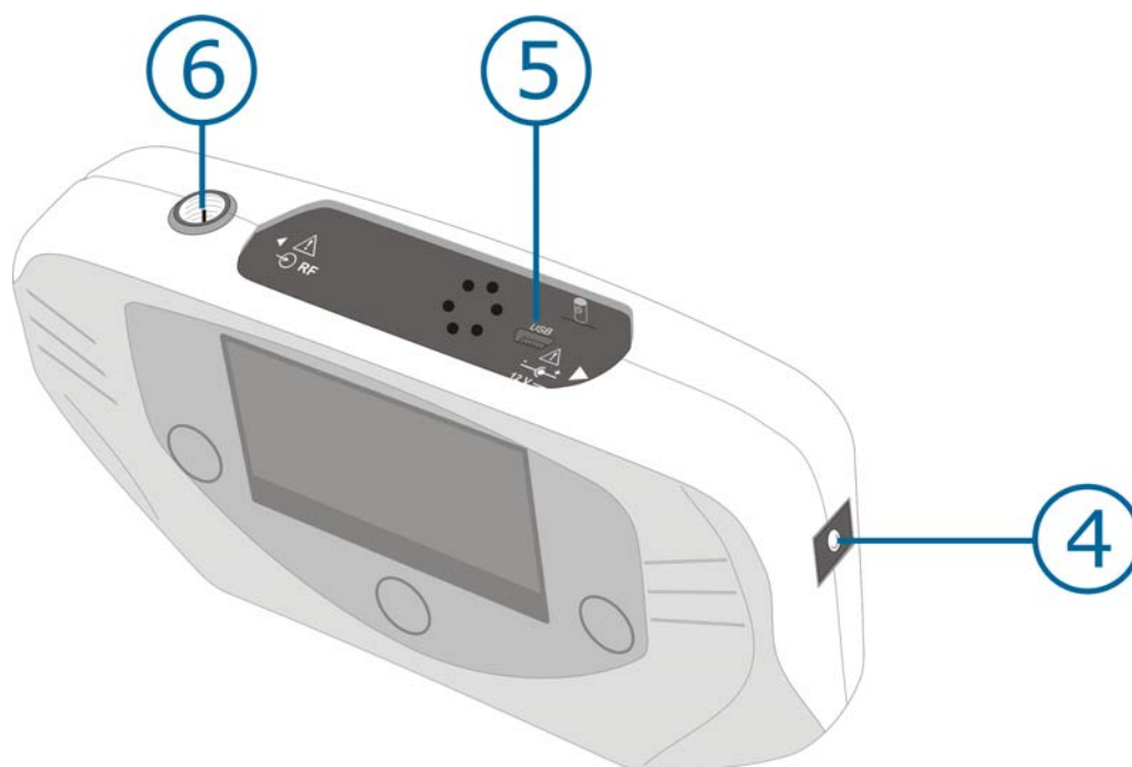
Figura 6. Paneles laterales.
