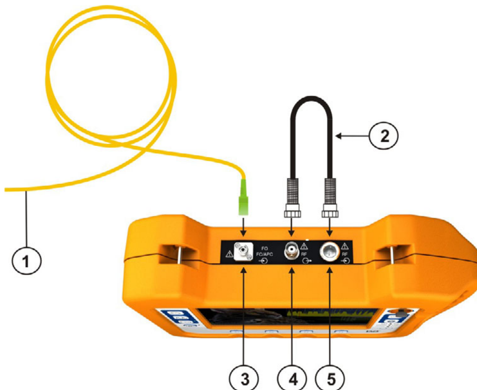
Рисунок A5.6. Верхняя панель HD RANGER 2 (с этой установленной опцией).
