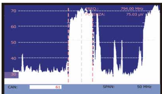
Figura 51.- Modalità Analizzatore di Spettri.
