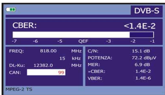
Figura 38.- Schermo di misura del CBER di segnali modulati in QPSK.
