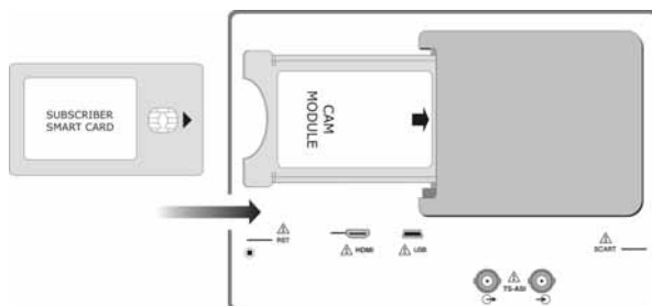
Figura 80.- Inserimento di un modulo CAM e scheda di abbonato (SMART-CARD).
