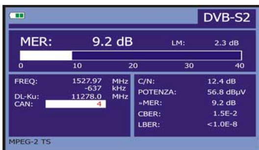
Figura 44.- Schermo di misura del MER per segnali DVB-S2 modulati in QPSK/8PSK.
