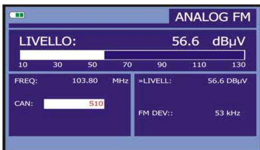
Figura 26.- Misura di livello segnale FM analogico.
