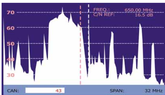
Figura 28.- Cursore NOISE. C/N (MANUALE).
