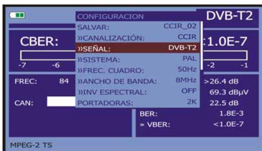
Figura 21 .- Configurazione schermata di misurazione dei segnali modulati COFDM.
