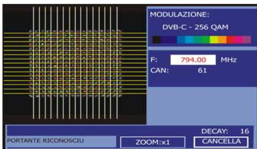
Figura 48.- Diagramma di costellazione. Segnale DVB-C (QAM 256).
