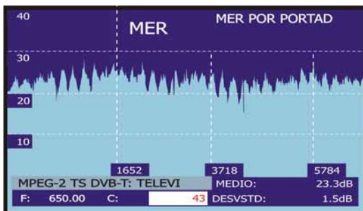
Figura 54.- Funzione MER da vettore.
