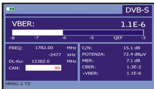
Figura 40.- Schermata di misura del VBER di segnali modulate in QPSK. (DVB-S).
