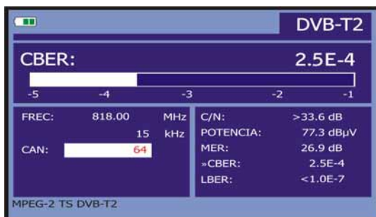
Figure 35.- CBER schermata di misurazione dei segnali modulati COFDM.
