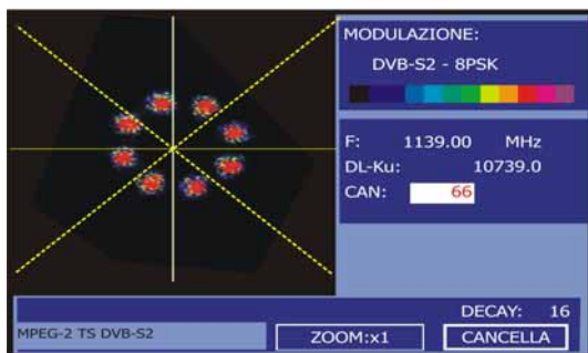
Figura 50.- Diagramma di costellazione. Segnale DVB-S2 (8PSK).
