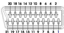
Figura 79.- Presa SCART (vista esterna).
