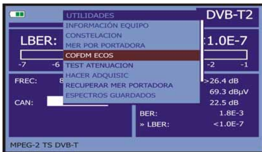
Figura 59.-. Menu COFDM ECHOES.
