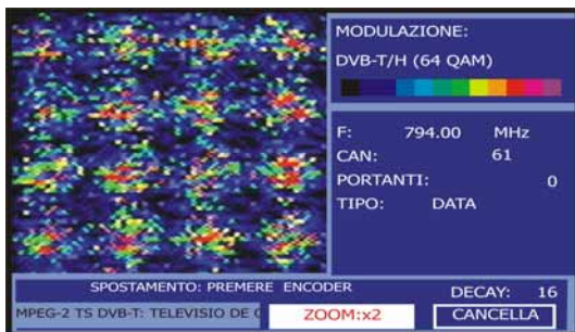
Figura 46.- Zoom x2 del diagramma di costellazione.
