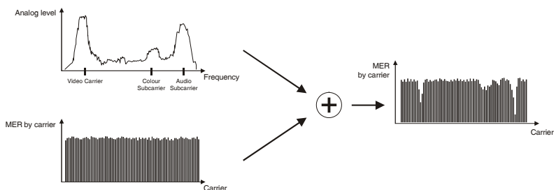
Figura 55.- Schema di interferenze del segnale analogico TV sui canali digitali.
