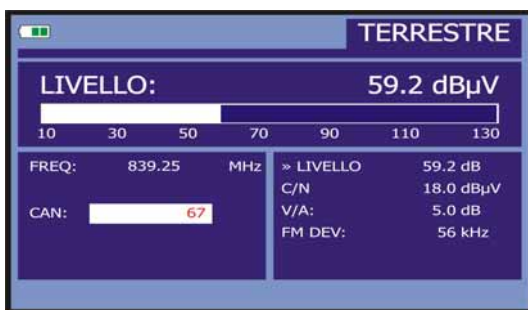
Figura 23.- Misura del livello di segnale analogico su banda terrestre.
