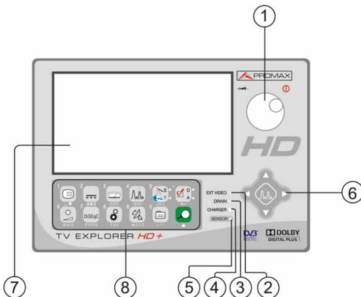
Figura 3.- Pannello frontale.
