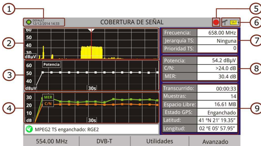
Figure 87. Cobertura de Señal de Canal Único
