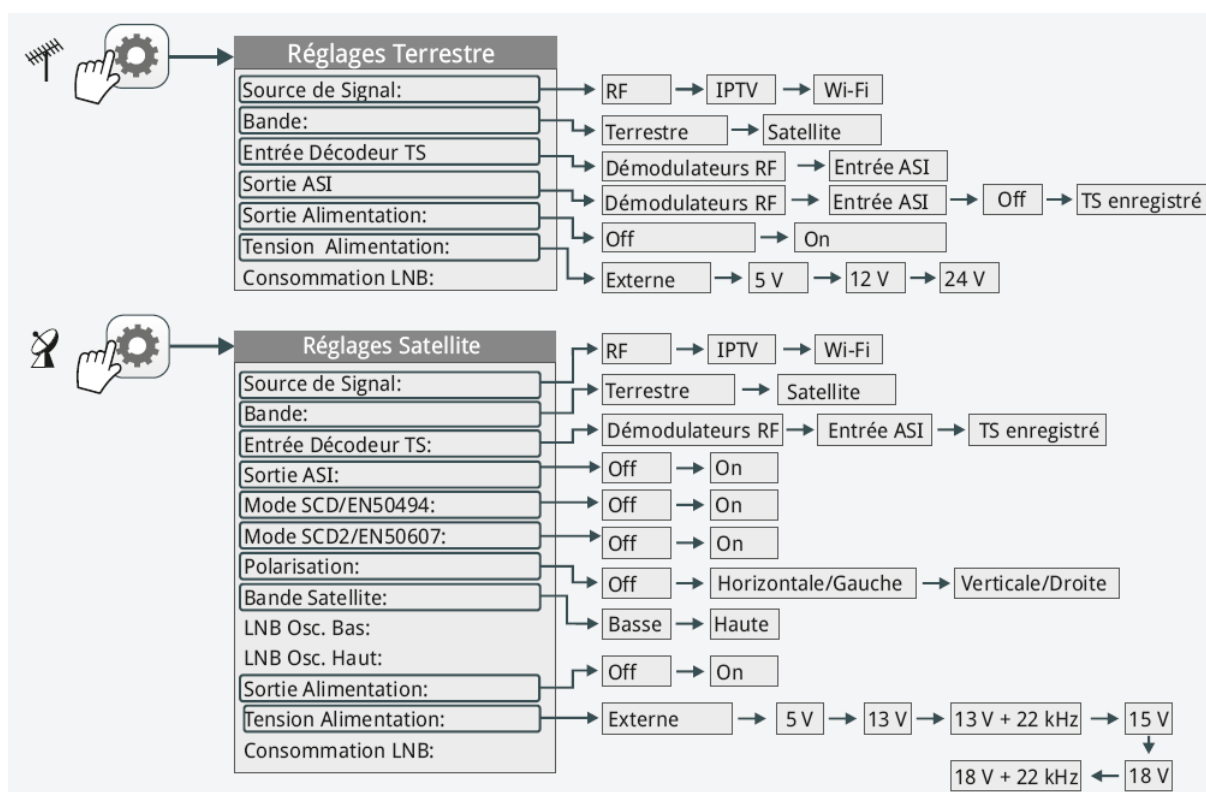
Figure 45. Réglages pour signaux RF (bande terrestre et satellite)
