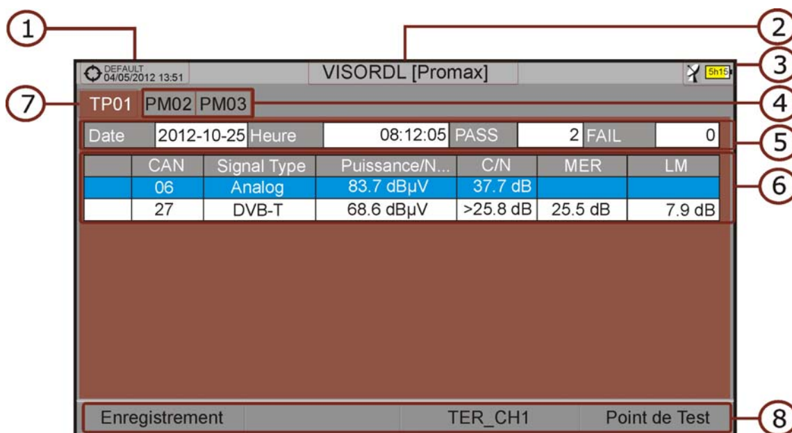
Figure 100. Visualisation du Datalogger d'un Plan de Fréquences.
