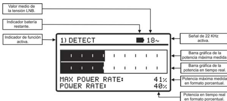
Figura 10.- Función DETECT.
