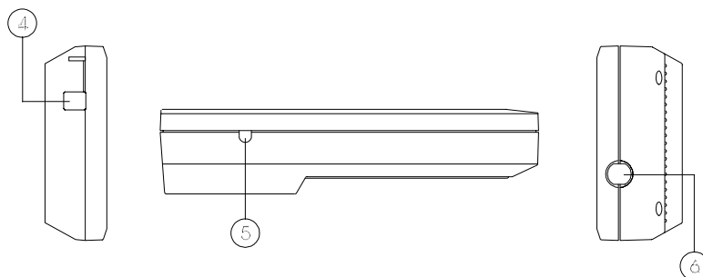
Figure 7.- Panneaux latéraux
