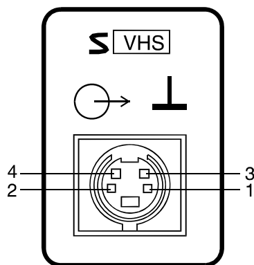
Figure 8.- Connecteur S-VHS
