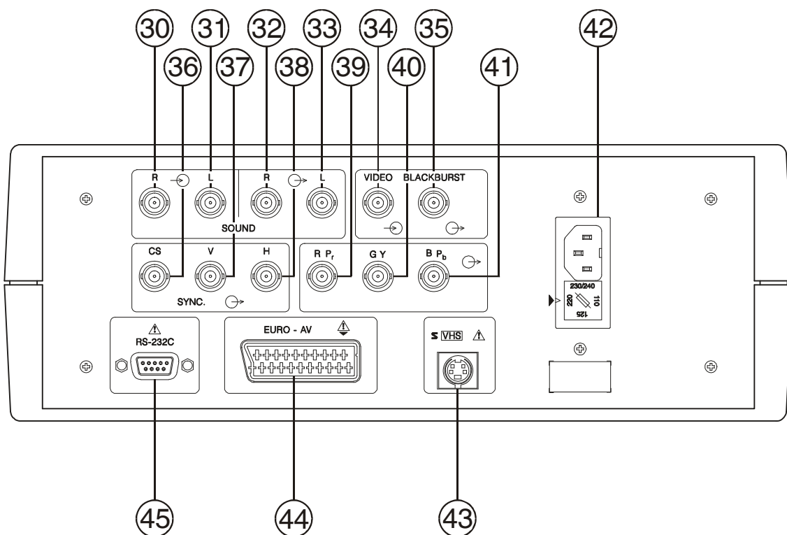
Figura 3.- Panel posterior
