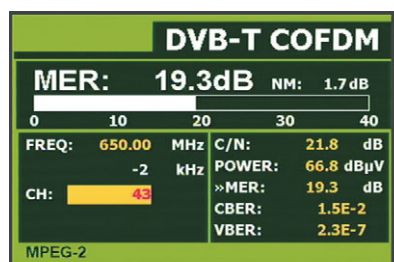
Muestra de una señal de test con datos PRBS
