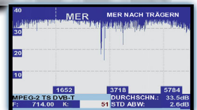
MER für jeden Träger bei DVB-T2 und DVB-T
