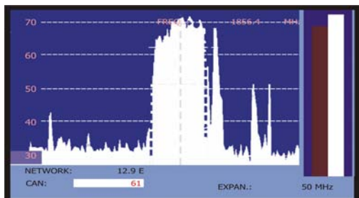
Figure 69.- Outil pour le pointage d'antennes.
