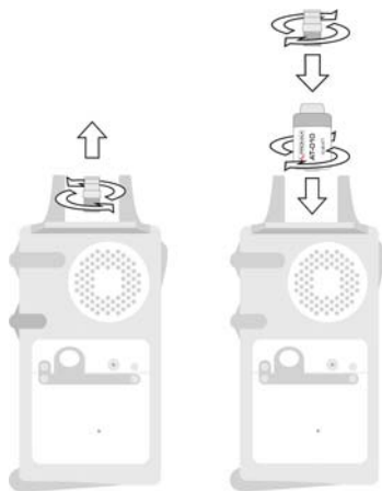
Figure 6.- Connexion de l'atténuateur externe à l'entrée RF [30].
