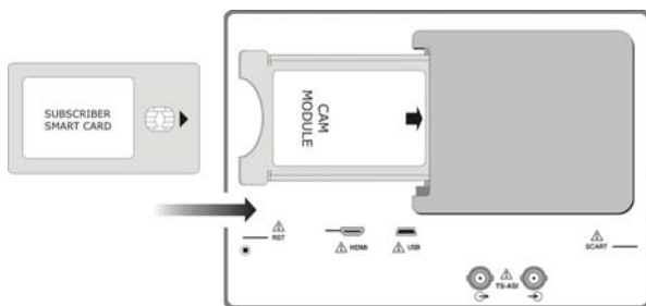
Figure 76.- Insertion d'un module CAM et carte d'abonné (SMART-CARD).
