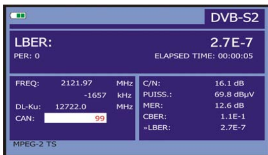
Figure 38.- Écran de mesure du LBER de signaux modulés en 8PSK. (DVB-S2).
