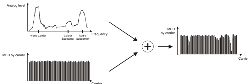
Figura 50.- Esquema de interferencia por señal TV analógica sobre canal digital.
