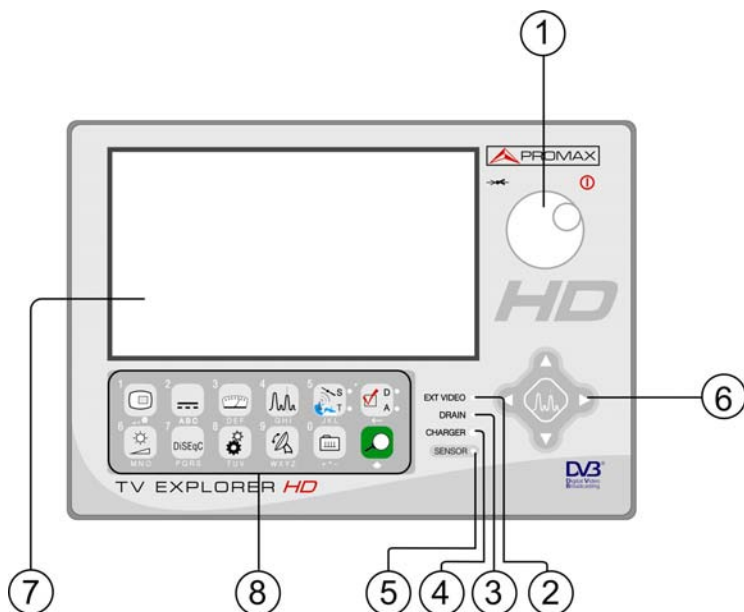
Figura 3.- Panel frontal.
