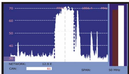
Figura 69.- Utilidad para el apuntamiento de antenas.
