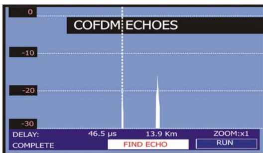
Figura 58.- ECHOES analysis.
