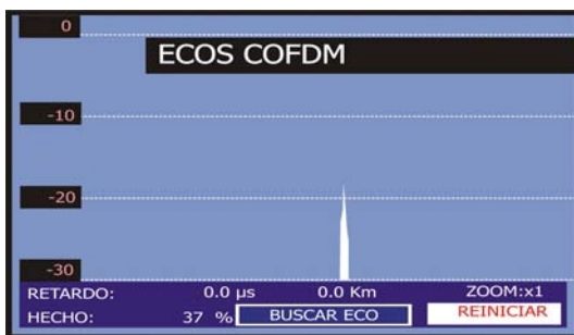
Figura 56.- Buscando ECOS.
