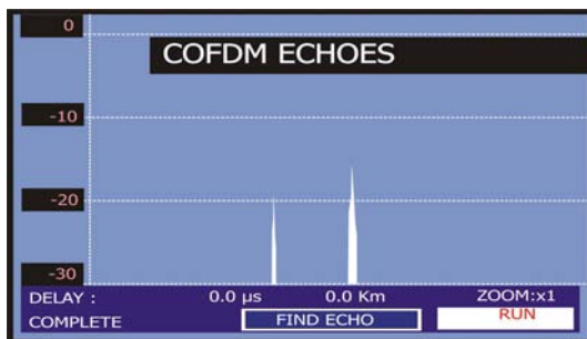
Figure 57.- ECHOS détectés.
