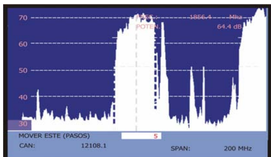
Figura 71.- Comandos DiSeqC: MOVER.
