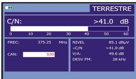
Figura 26.- Medida de la relación portadora/ruido (C/N).
