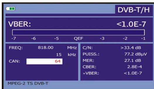
Figure 33.- Écran de mesure du BER de signaux modulés en COFDM. VBER.
