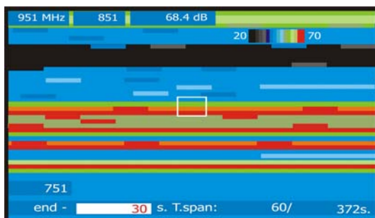
Figura 47.- Représentation du Spectrogramme.
