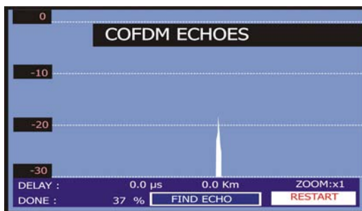
Figure 56.- Processus de détection des échos.
