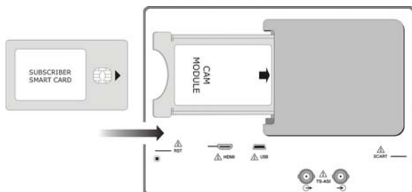
Figura 76.- Inserción de un módulo CAM y tarjeta de abonado (SMART-CARD).
