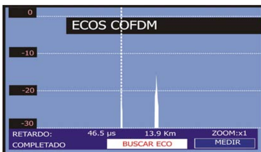
Figura 58.- Análisis de ECOS.
