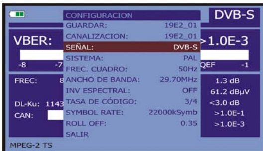
Figura 21.- Pantalla de configuración de medida de señales moduladas en QPSK .
