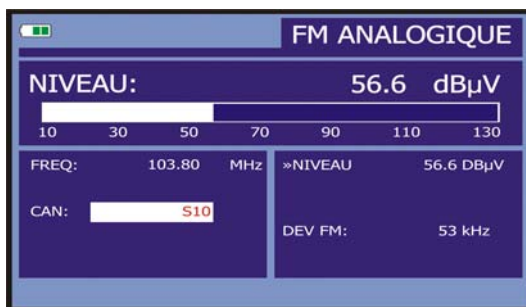
Figure 25.- Mesure du niveau de signal FM Analogique.
