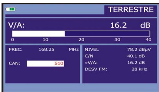
Figura 23.- Medida de la relación vídeo/audio.
