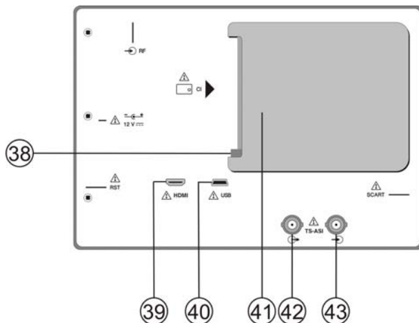
Figure 8.- Panneau postérieur.
