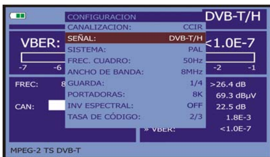
Figura 20.- Pantalla de configuración de medida de señales moduladas en COFDM .
