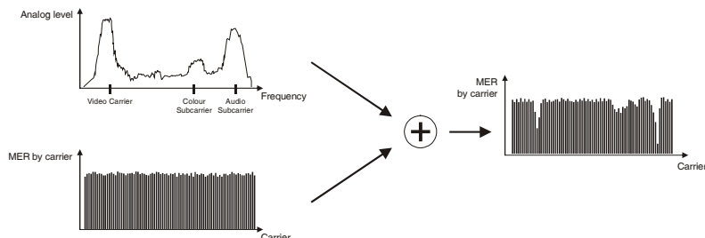
Figure 50.- Schéma d'interférence par signal TV analogique sur le canal numérique.
