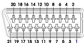
Figura 75.- Euroconector (vista externa).
