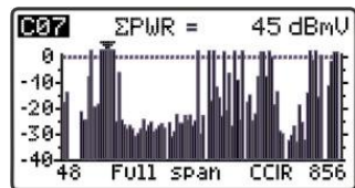
Figura 12.- Modo SCAN. función detección de potencia.
