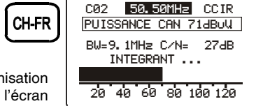
Figure 24.- Syntonie par fréquence.
