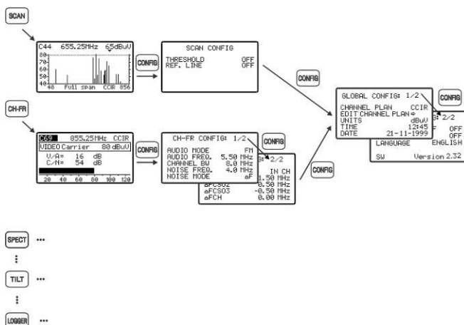
Figure 4.- L'accès au menu de configuration du PROMAX-8 SE .
