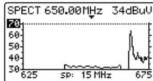
Figure 33.- Modification du niveau de référence
