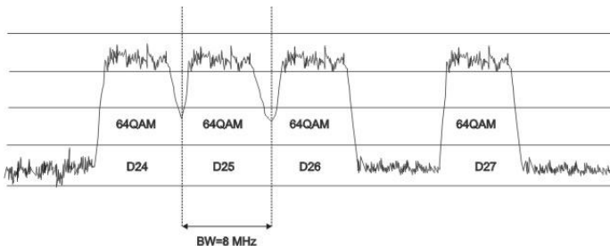
Figura 20.- Ejemplo de un espectro de canales digitales.
