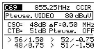
Figure 17.- Mesure CSO et CTB.
