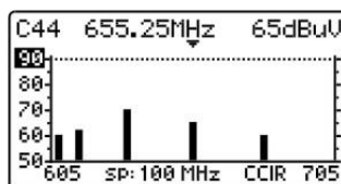
Figure 10.- Mode BALAI, Réf. 90 dB \mu V.
