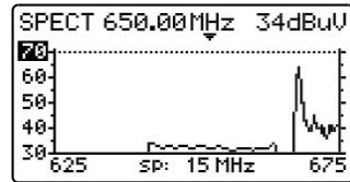
Figura 33.- Modificación del nivel de referencia.
