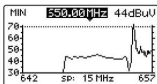
Figure 36.- Mode MIN. Première mesure.
