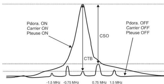
Figure 16.- Interprétation des mesures CSO et CTB.
