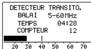
Figure 38.- Mode détecteur de transitoires.
