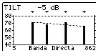
Figura 40.- Modo de operación TILT.
