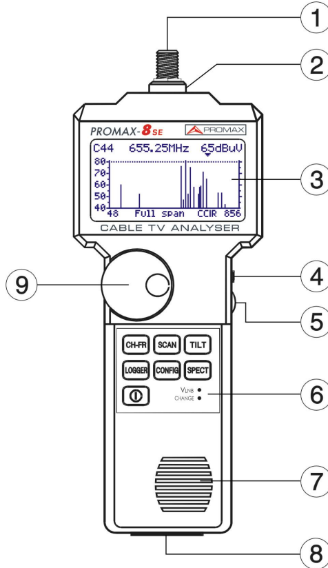
Figure 2.- Vue avant.
