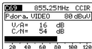
Figura 14.- Medida de nivel, V/A y C/N.
