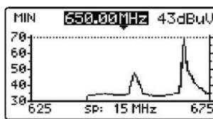
Figure 37.- Mode MIN. Après plusieurs mesures.
