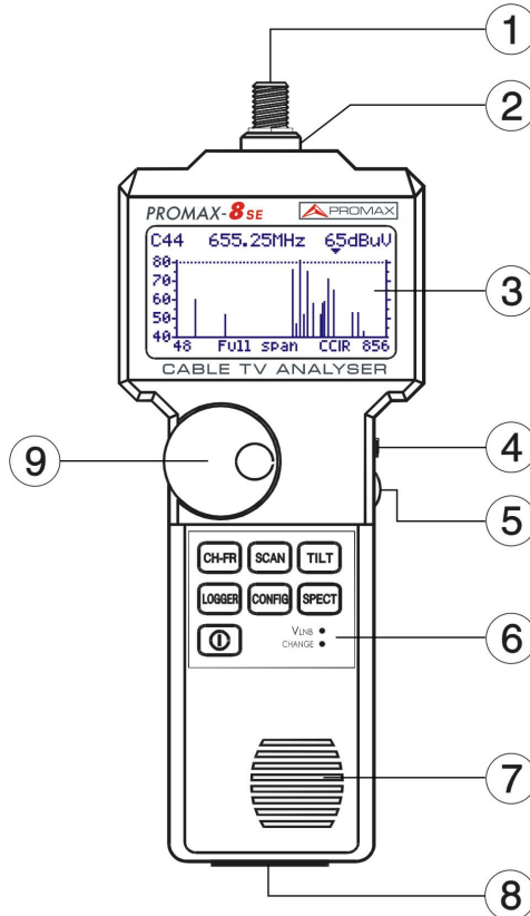
Figura 2.- Vista frontal
