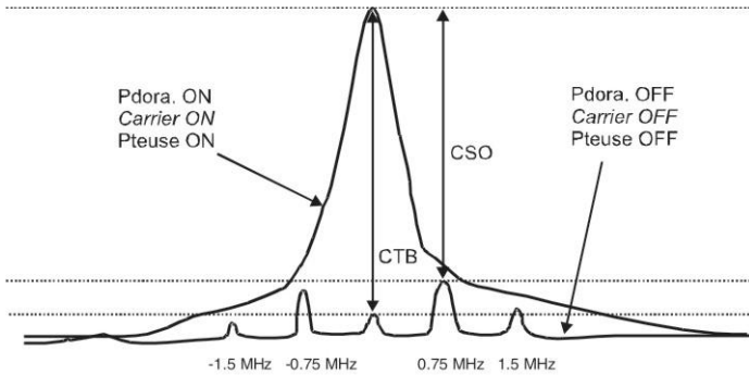
Figura 16.- Interpretación de las medidas CSO y CTB.
