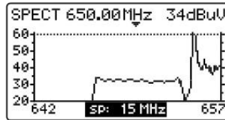
Figure 32.- Mode SPECT, réduction du span.
