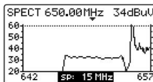
Figura 32.- Modo SPECT, reducción del span.
