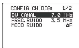
Figura 21.- Configuración para señales digitales en modo sintonía por canal.
