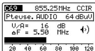
Figure 15.- Démodulation et mesure du signal de son.
