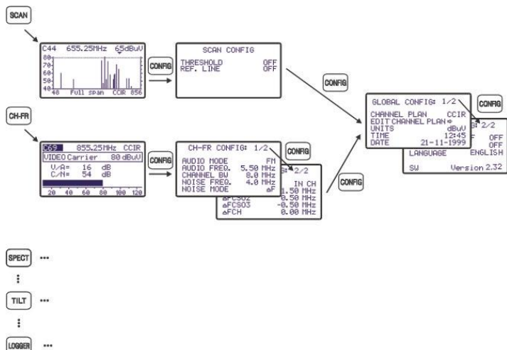
Figura 4.- Acceso a menús de configuración PROMAX-8 SE .
