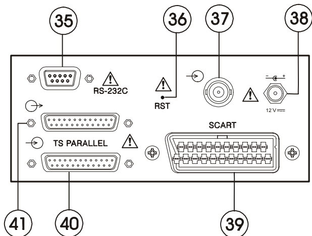
Figura 3.- Conectores del panel lateral.
