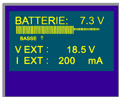
Figure 29.- Fonction Batterie & Lnb.
