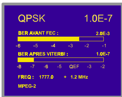
Figure 17.- Écran de mesure du BER des signaux modulés QPSK.
