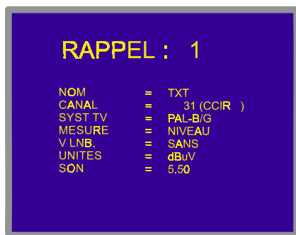
Figure 45.- Écran RAPPEL, récupération d'une configuration de mesure.
