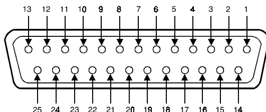
Figure 51.- Connecteur parallèle (LVDS D-25). Vue extérieure.
