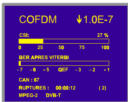
Figure 16.- Compteur RUPTURES. Dans l'exemple un total de 12 secondes sans MPEG-2 a été enregistré après 2 coupures.
