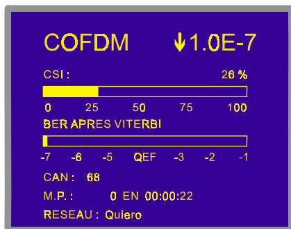
Figure 22.- Canal numérique syntonisé avec le niveau du BER acceptable.
