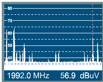
Figure 39.- Mode Analyseur de Spectres.
