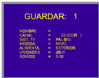
Figura 44.- Pantalla GUARDAR, almacenamiento de una configuración de medida.
