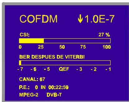
Figura 14.- Pantalla de medida del BER de señales moduladas en COFDM.
