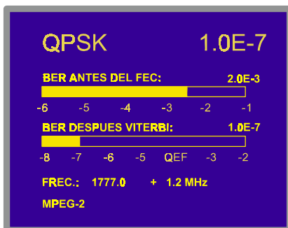
Figura 17.- Pantalla de medida del BER de señales moduladas en QPSK.
