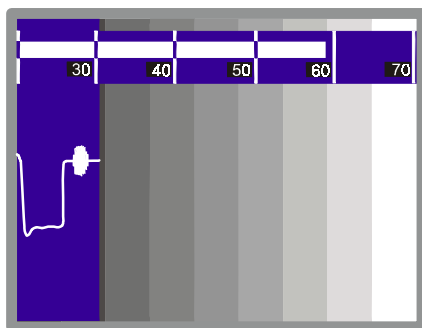
Figure 7.- Synchronisme + niveau + TV (TV+NV+SYNC)
