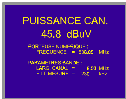
Figure 11.- Mesure de puissance des canaux numériques.
