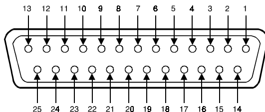
Figura 51.- Conector paralelo (LVDS D-25). Vista exterior.
