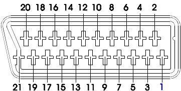
Figura 52.- Euroconector (vista exterior)
