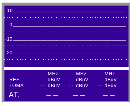
Figura 34.- Prueba FI Sat.
