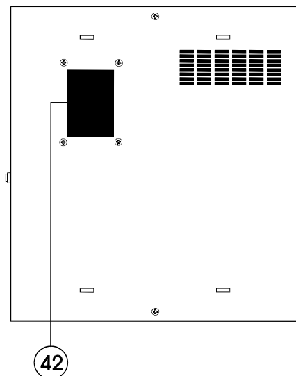
Figure 4.- Connecteur Smart-Card du panneau supérieur.
