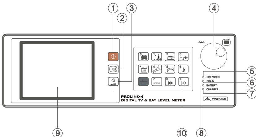
Figura 1.- Panel frontal.
