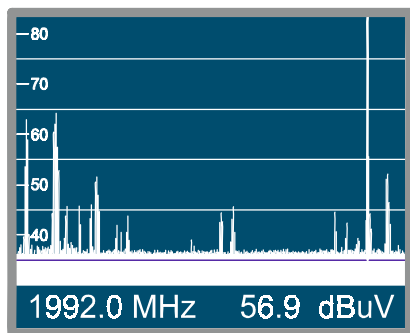
Figura 39.- Modo Analizador de Espectros
