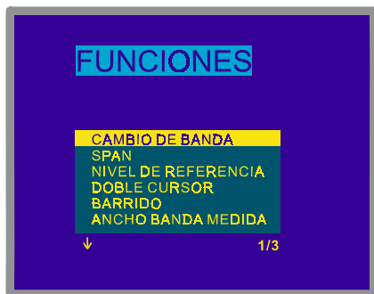
Figura 40.- Menú de funciones del modo Analizador de Espectros.
