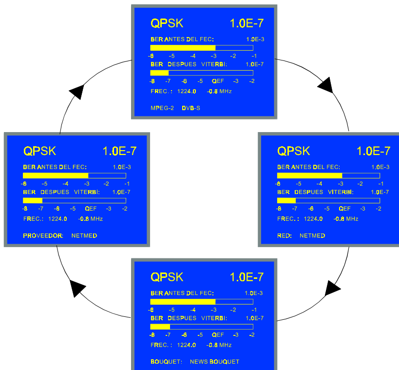
Figura 21.- Función DCI. En este ejemplo la información codificada por el operador en los campos Proveedor y Red es la misma.
