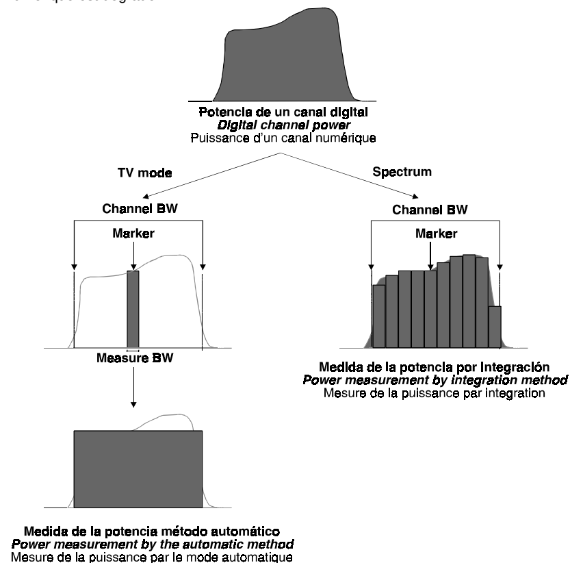
Figure 10.- Mesure de la puissance des canaux numériques.
