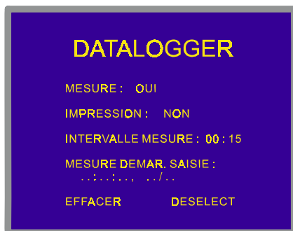
Figure 31.- Configuration de la fonction DATALOGGER
