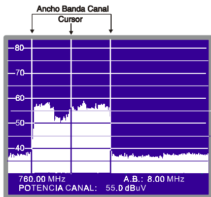
Figura 43.- Medida de la potencia de un canal en modo espectro.
