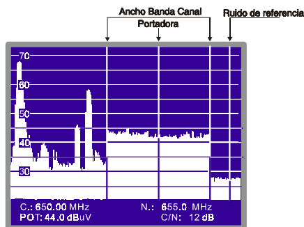
Figura 42.- Medida C/N en el modo Espectro (canal digital)
