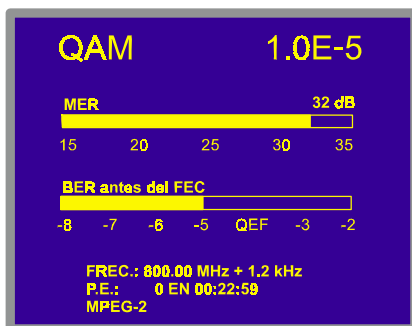
Figura 12.- Pantalla de medida del BER de señales moduladas en QAM.
