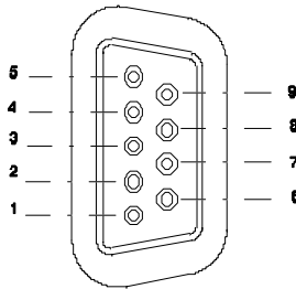
Figura 50.- Conector RS-232C. Vista exterior.
