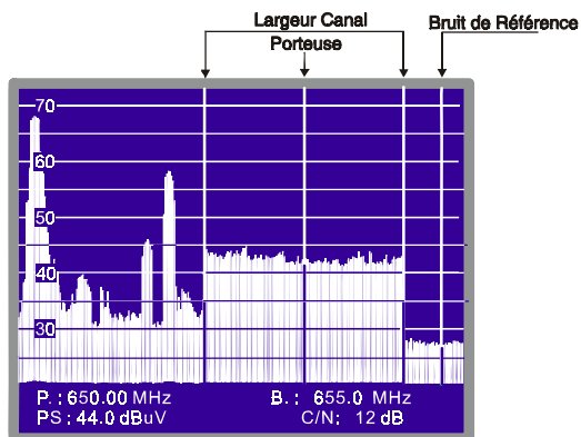
Figure 42.- Mesure C/N dans le mode Spectre (canal numérique).
