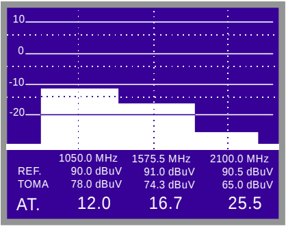
Figura 36.- Medidas de atenuación para una toma.
