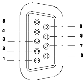
Figure 50.- Connecteur RS-232C. Raccordements vus de face.
