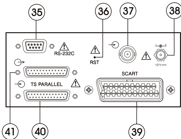
Figure 3.- Connecteurs du panneau latéral.
