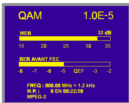
Figure 12.- Écran de mesure du BER des signaux modulés en QAM.
