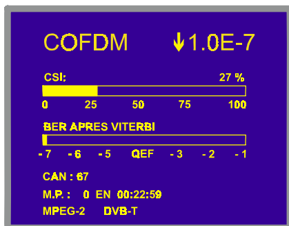
Figure 14.- Écran de mesure du BER des signaux modulés COFDM.
