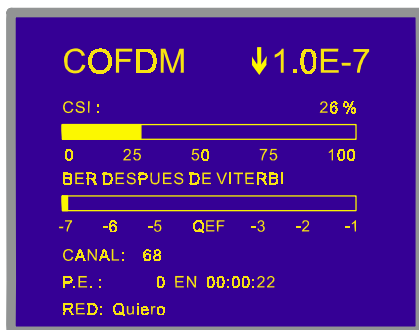
Figura 22.- Sintonización de un canal digital con nivel de BER aceptable.
