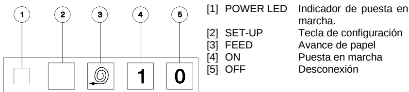
Figura 48.- Teclado impresora CI-23
