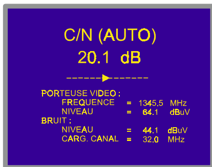
Figure 9.- Mesure du rapport porteuse / bruit C/N (mode Auto).
