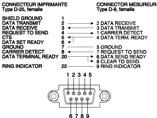
Figure 47.- PROLINK-4 connecteur RS-232C. Numération des pins.
