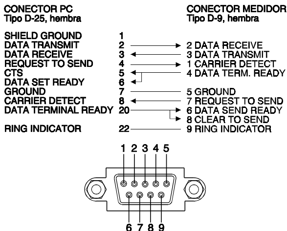
Figura 47.- Conector RS-232C PROLINK-4 . Numeración de los pins.
