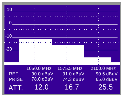
Figure 36.- Mesures d'atténuation pour une prise.
