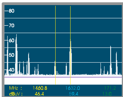
Figura 41.- Modo Analizador de Espectros con dos marcadores de sintonía.
