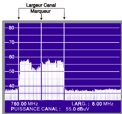
Figure 43.- Mesure de la puissance d'un canal en mode spectre.
