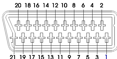
Figure 52.- Prise péritel
