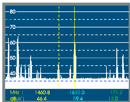
Figure 41.- Mode Analyseur de Spectres avec deux marqueurs de syntonie.
