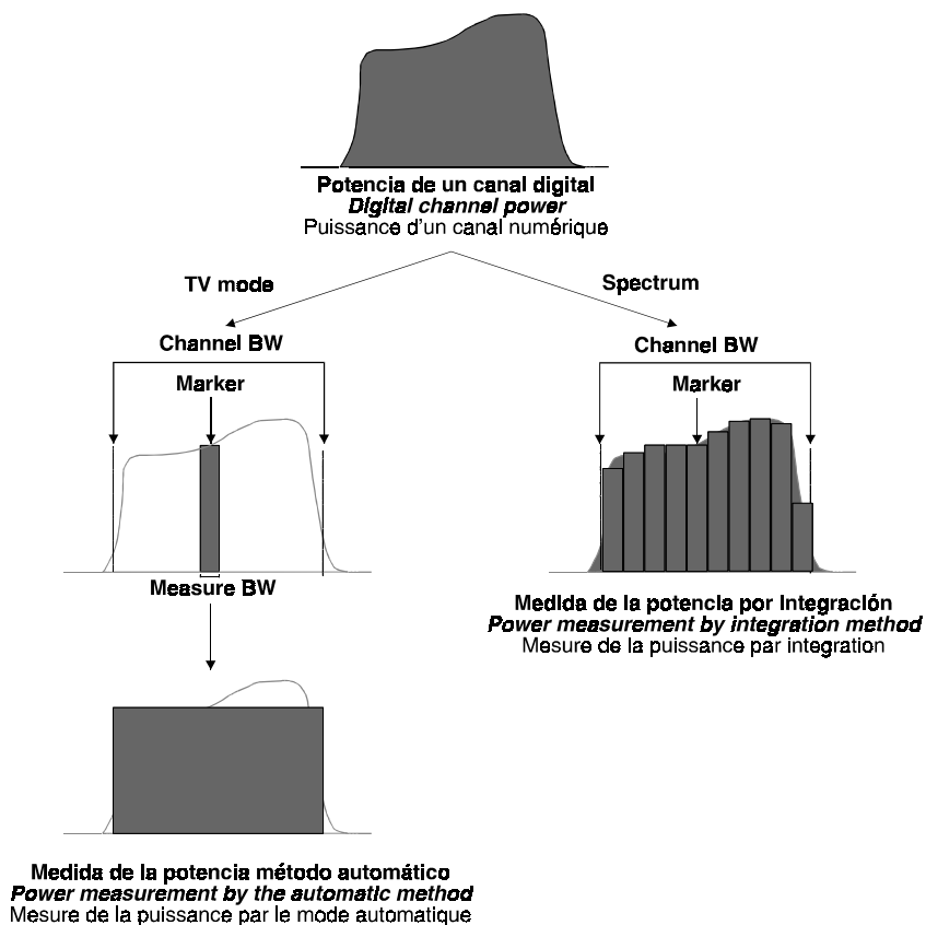
Figura 10.- Medida de la potencia de una señal digital.
