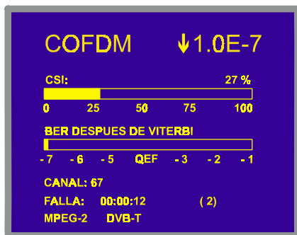
Figura 16.- Señalización de 2 cortes en la recepción de la señal MPEG con una duración total de 12 segundos.
