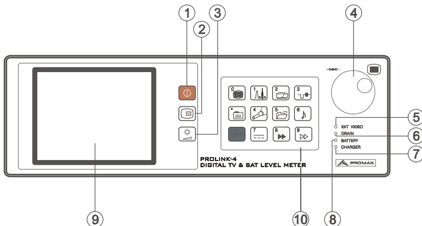
Figure 1.- Panneau avant
