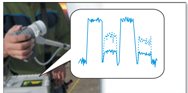
Ajuste de la polarización cruzada rotando el LNB
