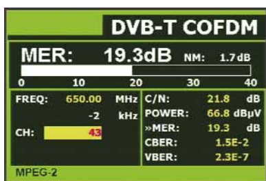
Messung eines vom MO-170 ohne externen Transport Stream erzeugten Signals
