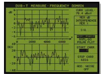
Amplitude und Phase des fixen Rice-Kanals F1 simuliert mit dem MO-170
