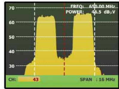
Lücke im Spektrum zeigt vorhandene Intermodulationsprodukte im Kanal
